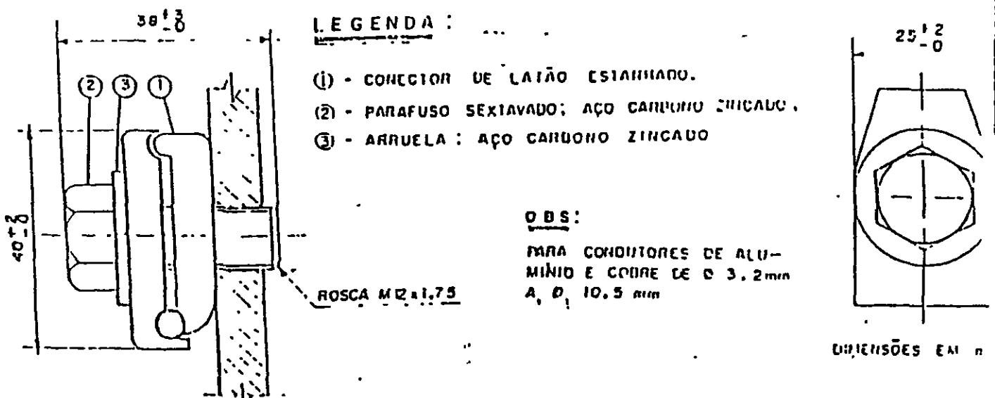
DISPOSITIVO DE ATERRAMENTO EM TRANSFORMADORES ATÉ 300 KVA
