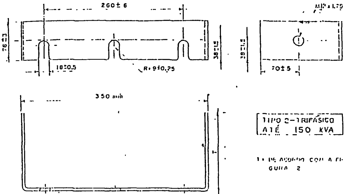
SUPORTE PARA FIXAÇÃO DO TRANSFORMADOR NO POSTE
